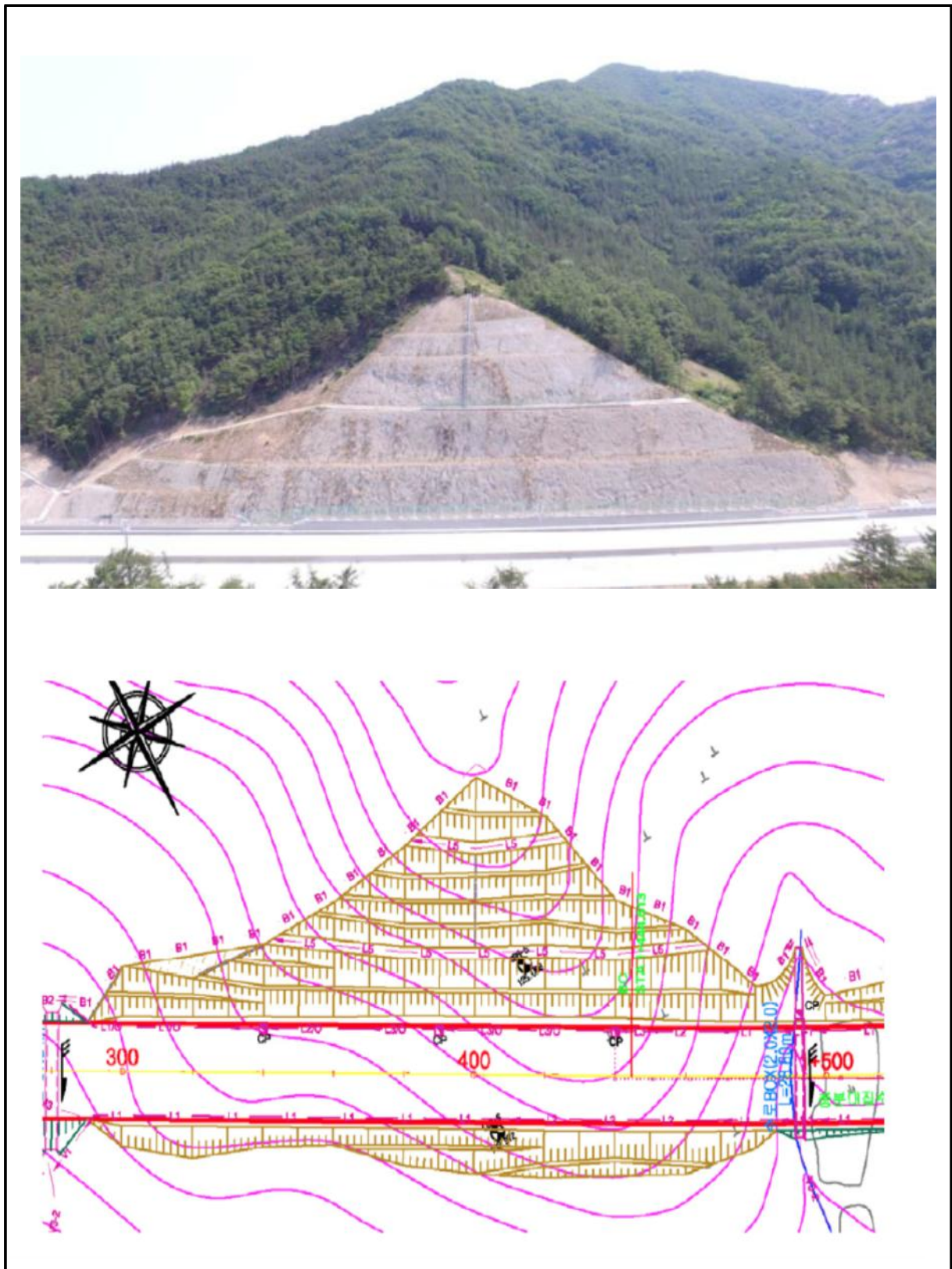
【그림 14.14】 상주절토14 검토대상 비탈면구간
