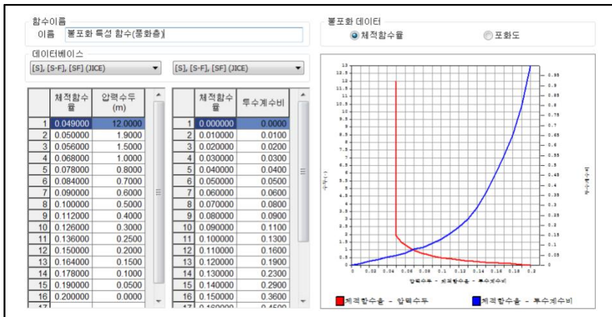
【그림 14.15】 압력수두-채적함수(포화도)-투수계수비 함수
